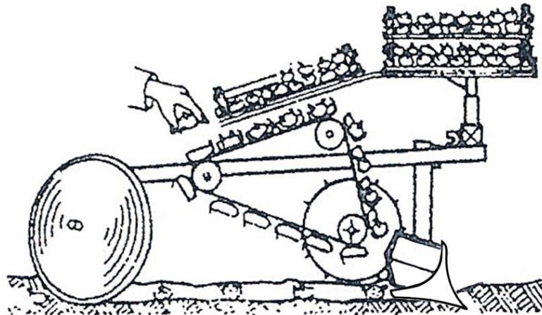
Slika 6. Poluautomatska sadilica krumpira s beskonačnom trakom
