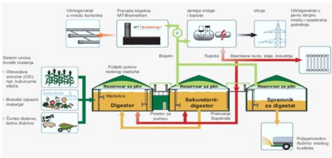
Slika 17. Predložena shema postrojenja za plin
