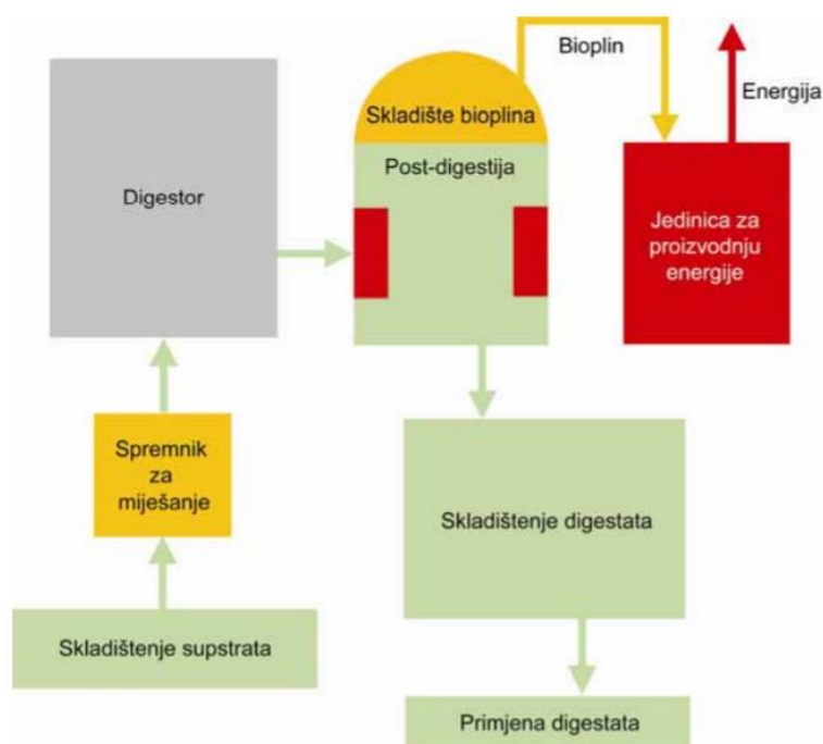
Slika 10. Glavni dijelovi postrojenja za proizvodnju bioplina
